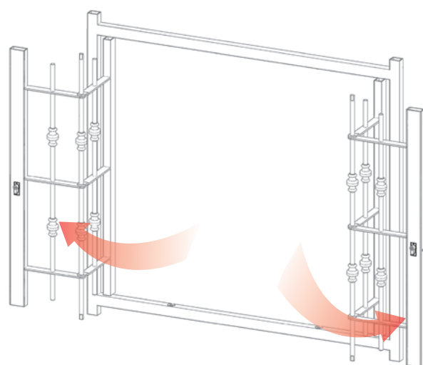
Ante aperte ribaltate sul serramento esterno per fare scomparire tutti gli scomodi ingombri. Open grille folded back against the exterior shutters in a totally unobstructive way.
