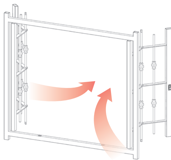
Grata aperta totalmente all'interno dell'abitazione per agevolare la chiusura della persiana o antone. Grille totally opened inwards to make it easier to close the exterior shutters.
