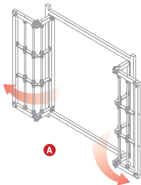
Ante aperte ribaltate sul serramento esterno per fare scomparire tutti gli scomodi ingombri. Open grille folded back against the exterior shutters in a totally unobstructive way.
